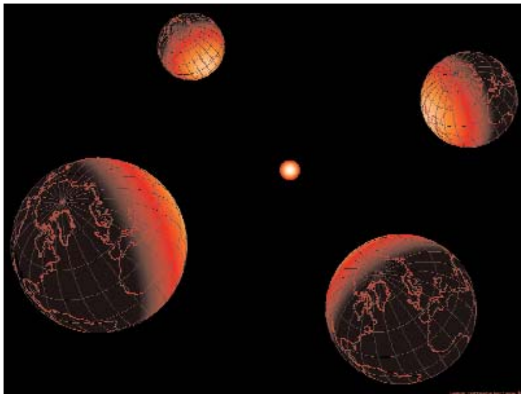
Posizion de Tiere ai solstizis (a drete e a çampe) e ai ecuinoziis (in alt e in bas)
